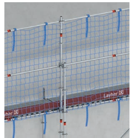
Roof edge protection
